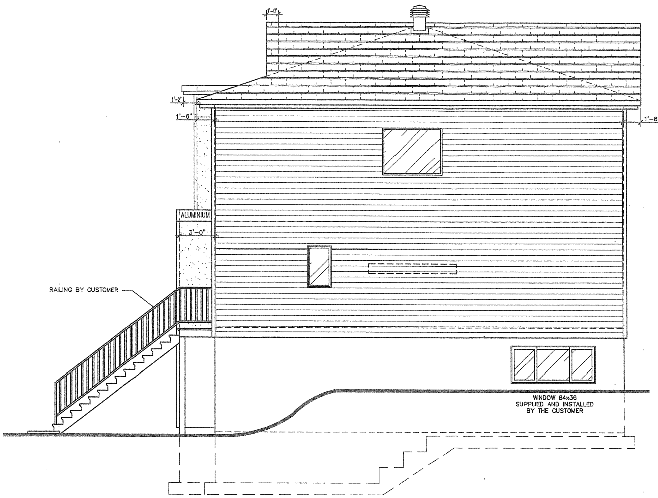
RIGHT ELEVATION
